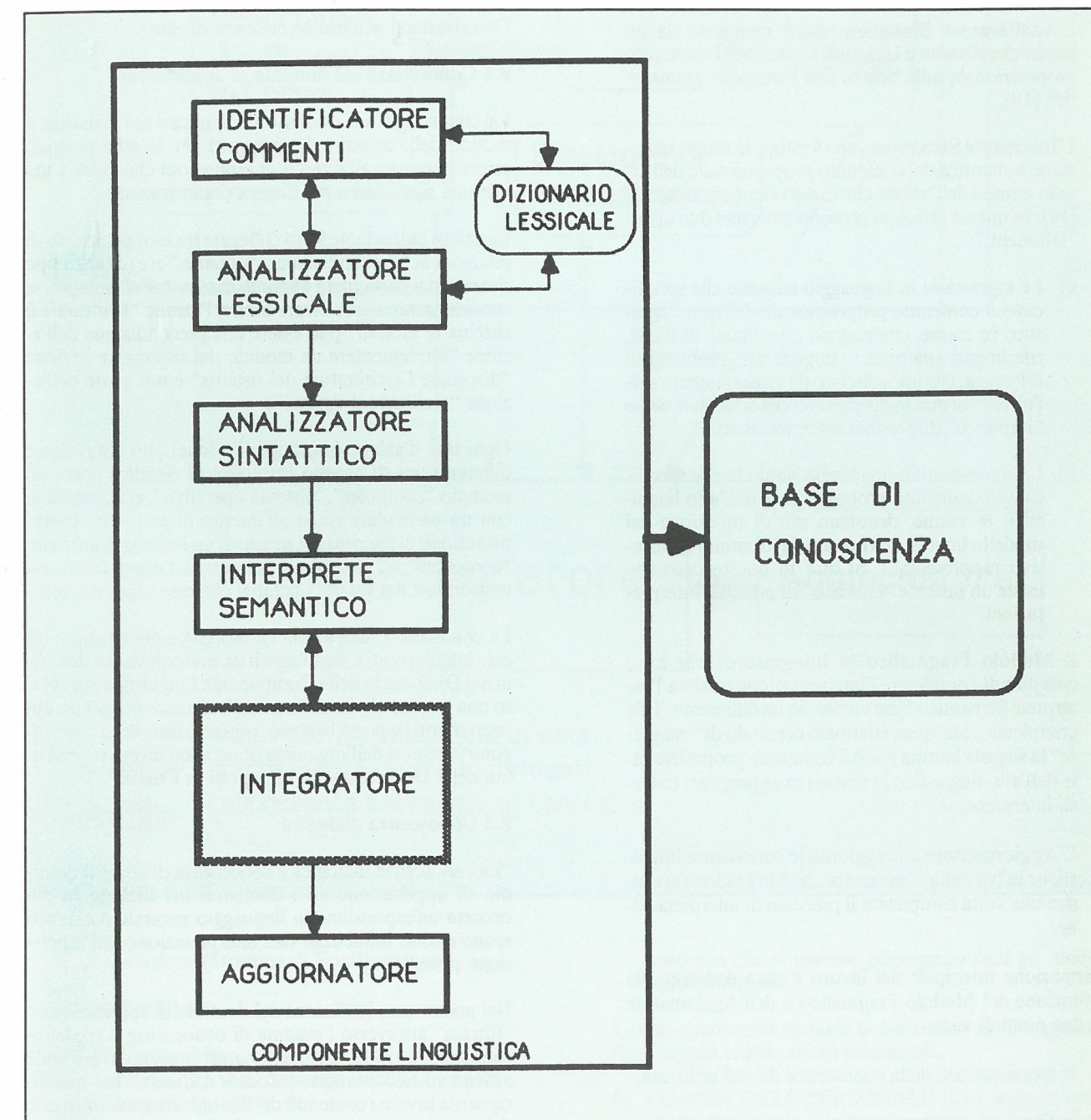
Fig. 5 La Componente Linguistica di Chaos2.
